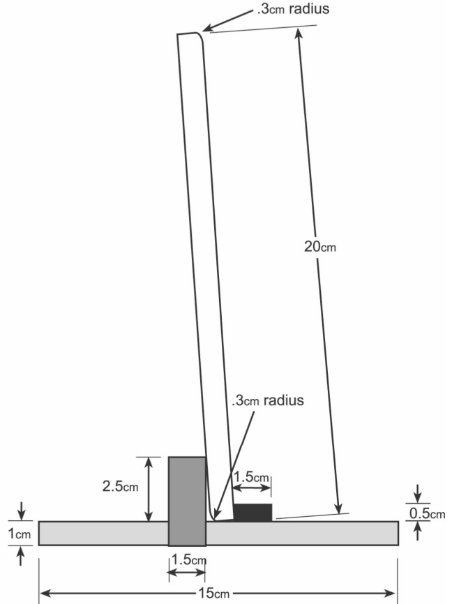
Πλήρης Στόχος Πλάγια Όψη
