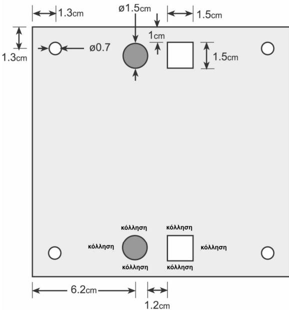
Βάση Στόχου (σχέδιο)
